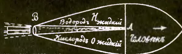
Схема межпланетного корабля из труда К. Э. Циолковского «Исследование мировых пространств реактивными приборами» (1903—1926 гг.).
